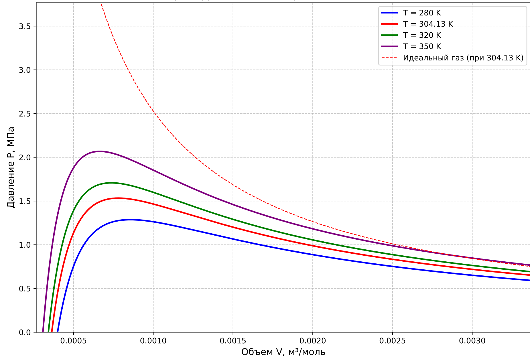
Изотермы уравнения Камерлинг-Оннеса для \text{CO}_2
